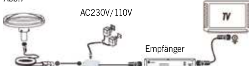
Installation 2: Verbindung durch den Empfänger (Abb. 7)
