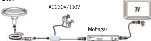
Installation 2: Ansluts via mottagar (Bild7)
