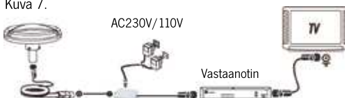
Asennus 2: Asennus vastaanottimen kautta (Kuva 7)
