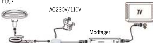
Installation 2: Forbindelse via modtageren (fig. 7)
