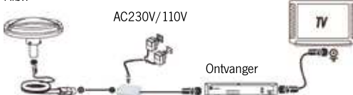
Installatie 2: Verbinding door ontvanger (Afb. 7)
